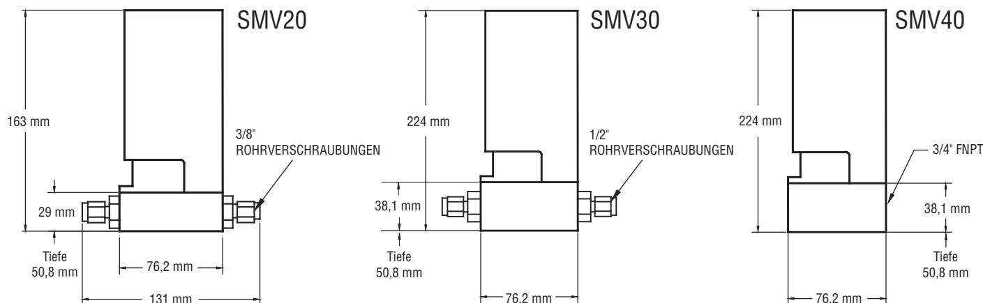
Abmessungen Schrittmotorventile
